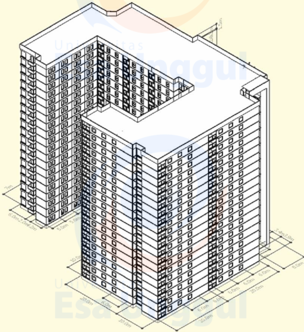
TAMPAK DEPAN BESERTA UKURAN DESAIN BANGUNAN VERTIKAL
